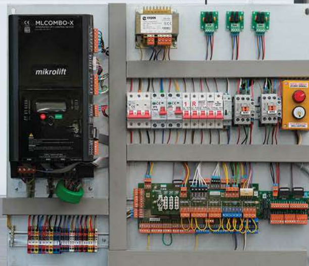
Dışlılı Pano (MR) Geared Control Panel (MR)
